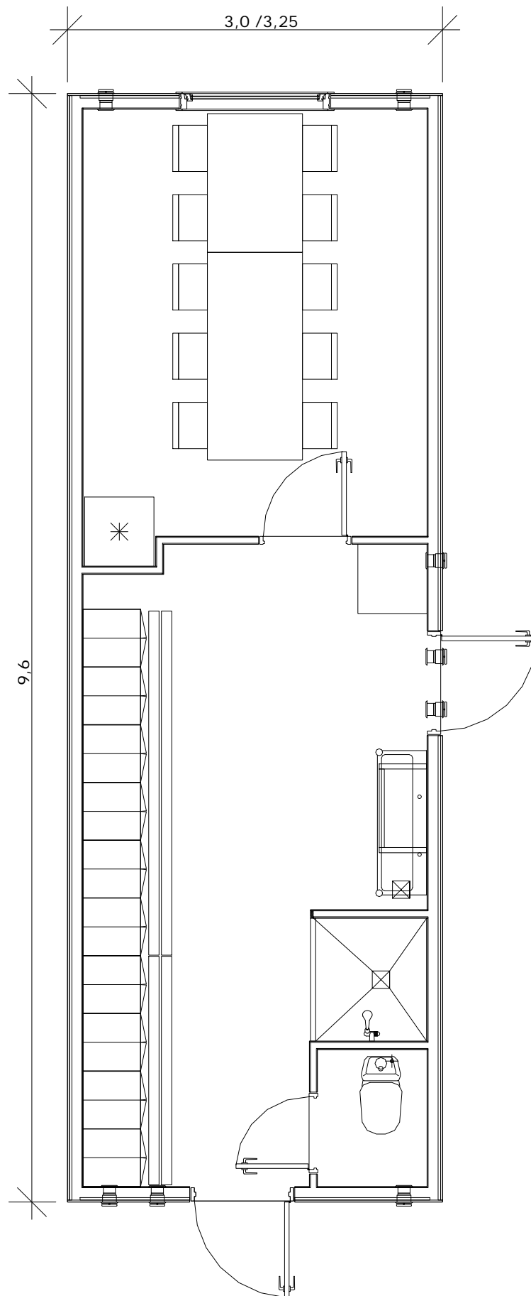
B-MS 10-30/33 MANDSKABSMODUL-BASIC
