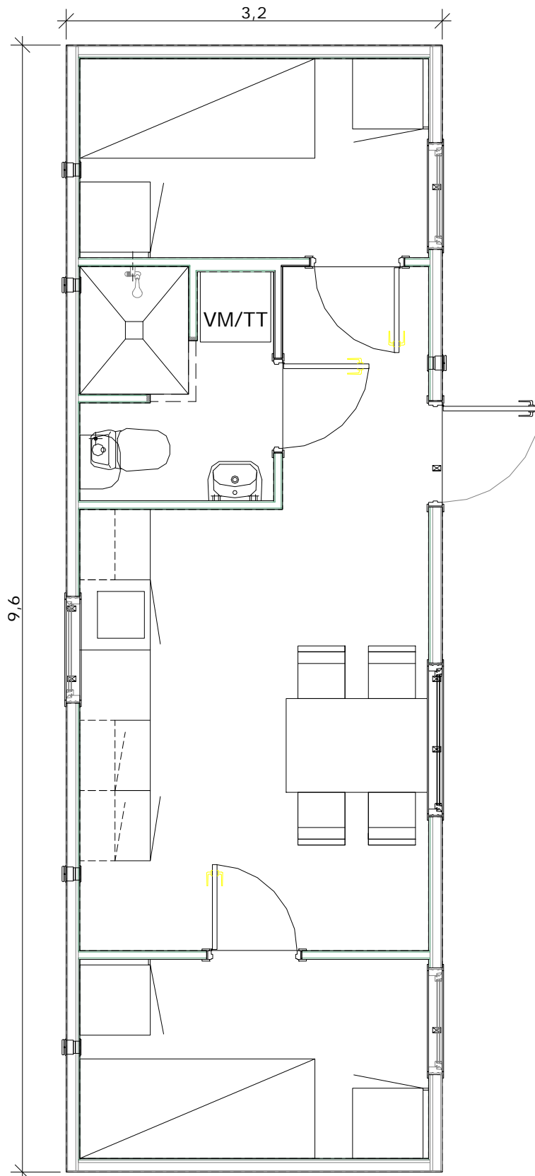
B-B 96-33 Beboelsesmodul
