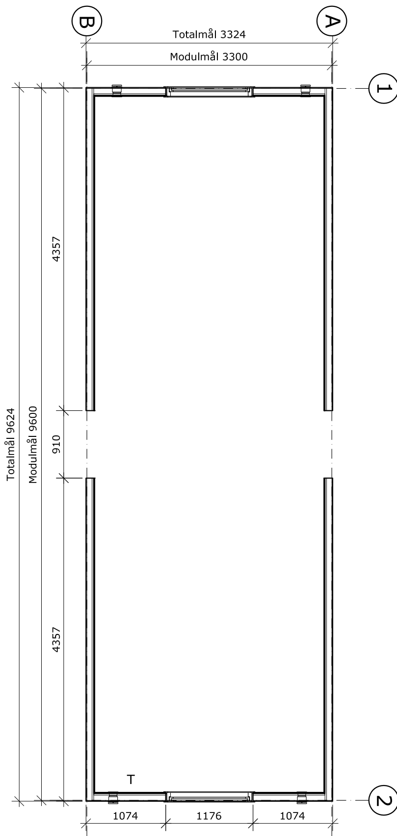
C-KM-C Kontormodul
